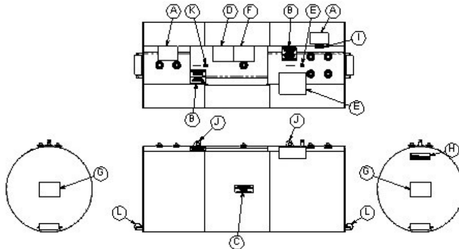
RÉSERVOIR CYLINDRIQUE, RECTAGULAIRE ET OBLONG/ CYLINDRICAL, RECTAGULAR AND OBROUND TANK
