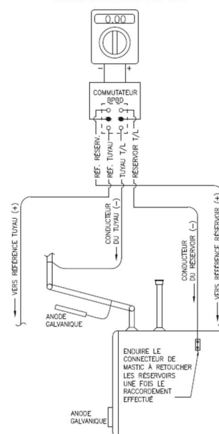
BORNE DE SURVEILLANCE À DISTANCE TYPE AVEC MULTIMÈTRE NUMÉRIQUE
